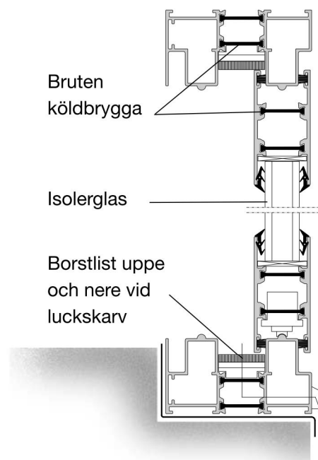
Vertikalt snitt
