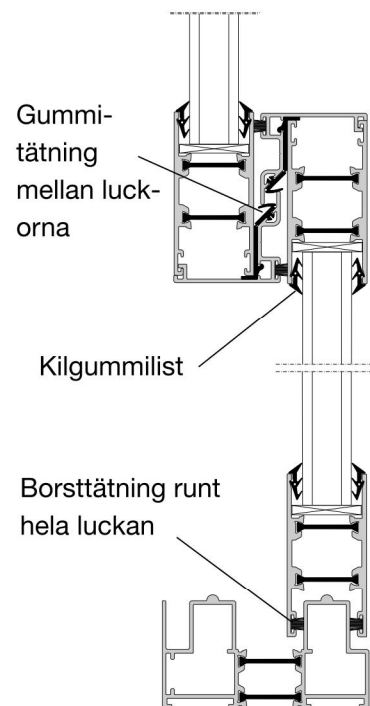
Horisontellt snitt
